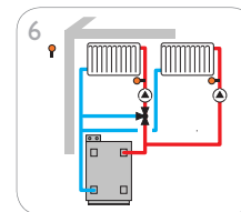
6 Een gemengd en een niet-gemengd verwarmingcircuit
