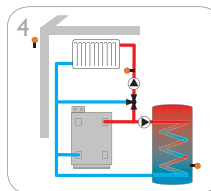
4 Een gemengd verwarmingcircuit met sanitair warmwaterbereiding
