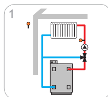
1 Een gemengd verwarmingcircuit
