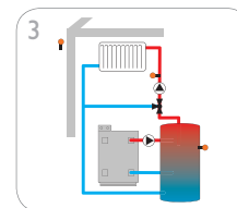
3 Een gemengd verwarmingcircuit met naverwarming en oplaadpomp
