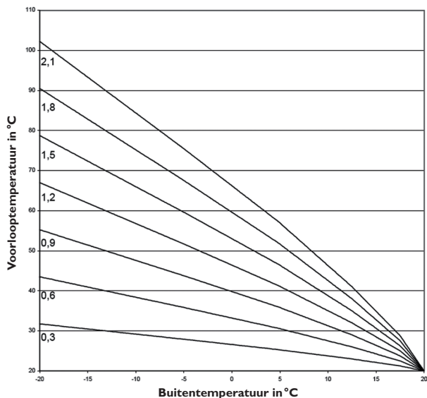
Verwarmingskarakteristieken
