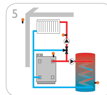
5 Een gemengd verwarmingcircuit met sanitair warmwaterbereiding en naverwarming
