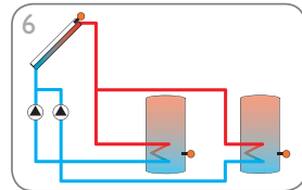
Zonne-energiesysteem met 2 boilers en pomplogica (pagina 13)
