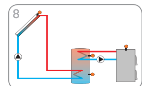
Zonne-energiesysteem met 1 boiler en vaste brandstofketel (pagina 16)
