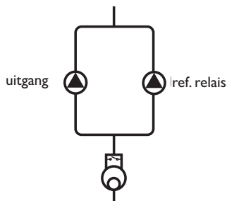
Voorbeeldschema voor tweelingpompen in de zonne-energieaanvoer met voorgeschakeld volumemeetgedeelte
