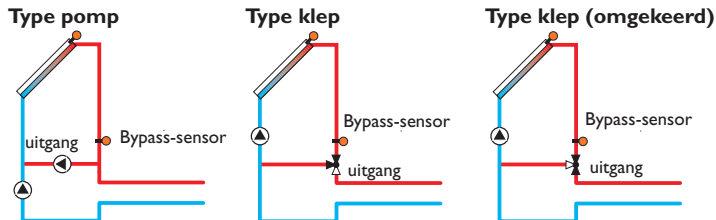
Voorbeeldschema's voor de verschillende bypass-uitvoeringen
